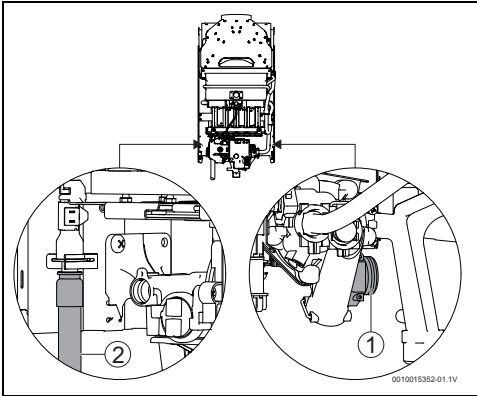
Bild 14 Wasseranschluss
