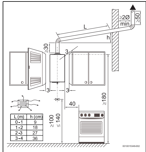
Bild 9 Mindestabstände (cm)
