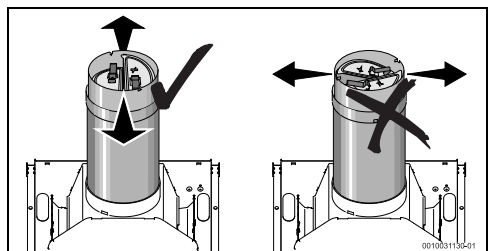
Bild 10 Abgasklappe montieren
